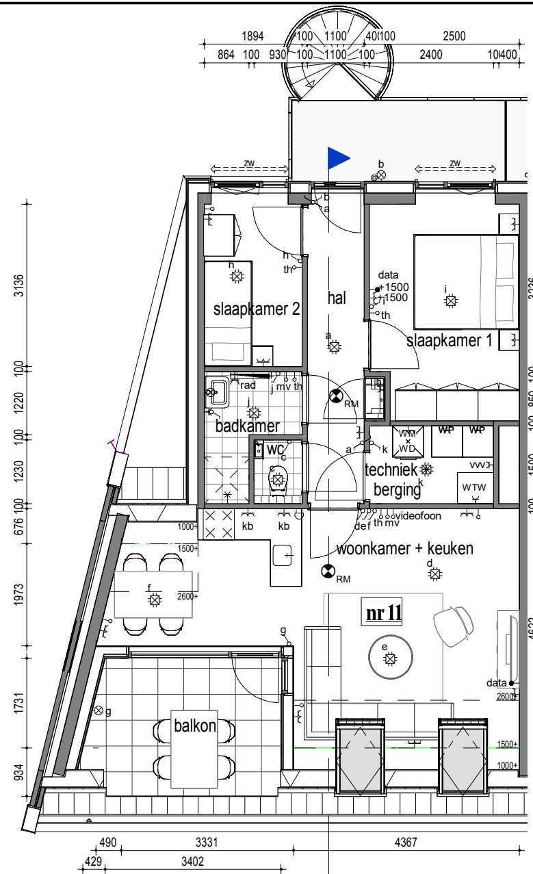
Plattegrond 1:100
