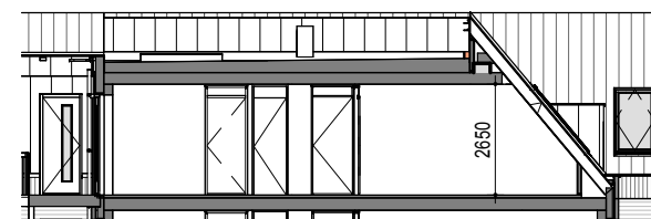
Doorsnede 1:200
