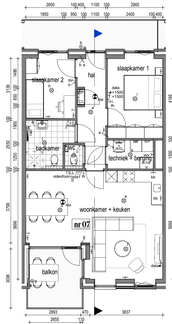
Plattegrond 1:100
