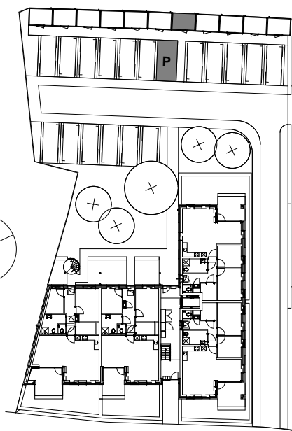
Situatie 1:1000
