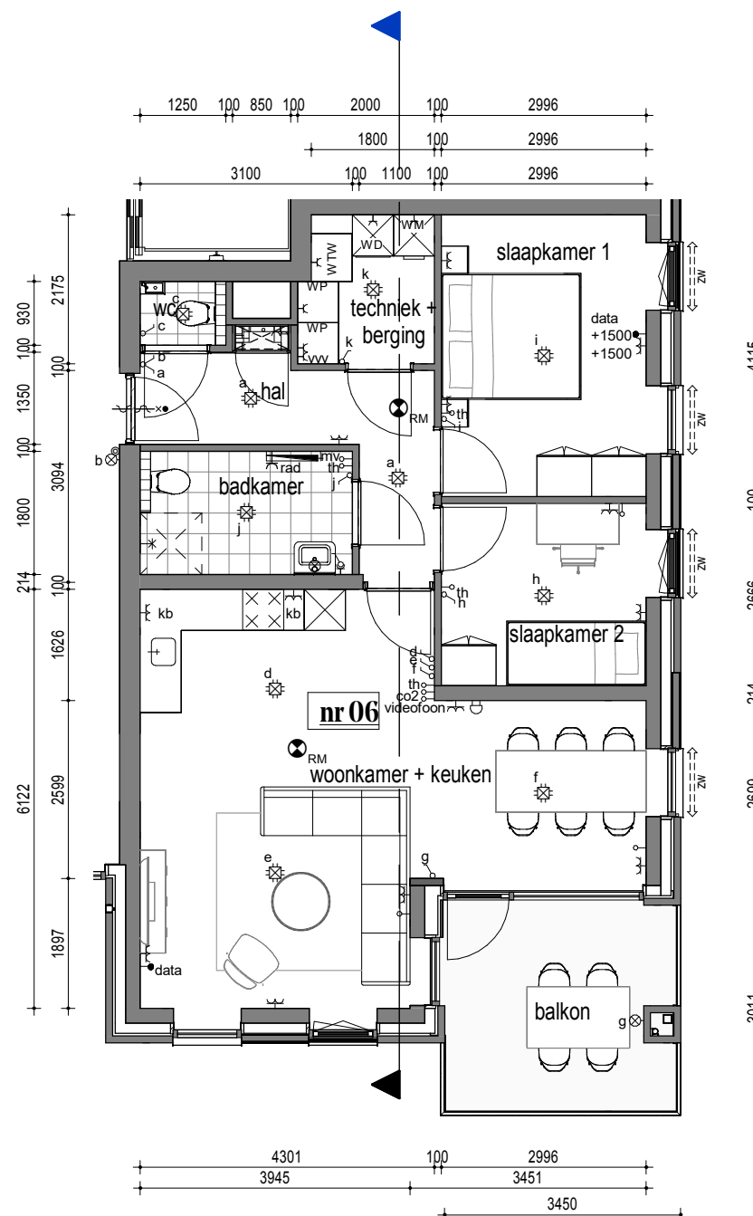
Plattegrond 1:100
