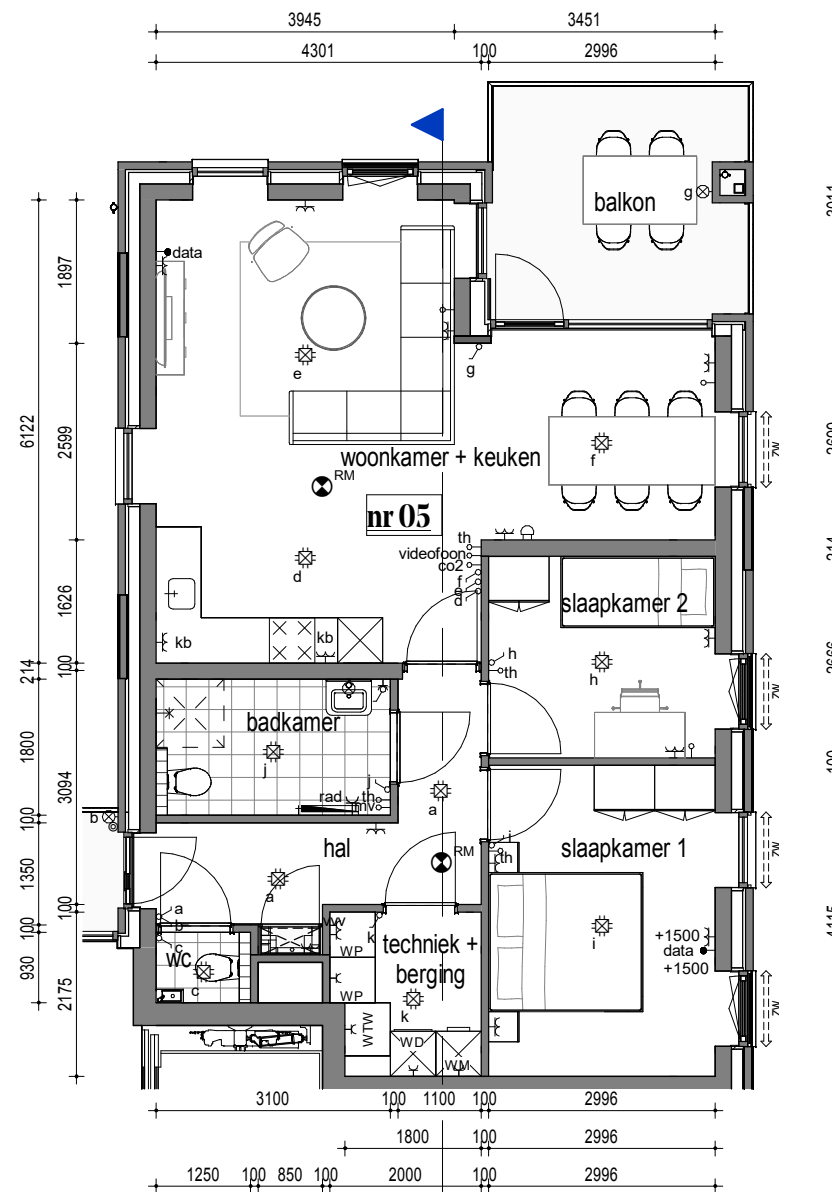
Plattegrond 1:100
