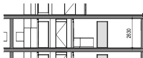
Doorsnede 1:200
