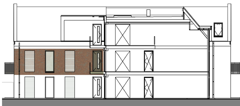
Linker zijgevel 1:250
