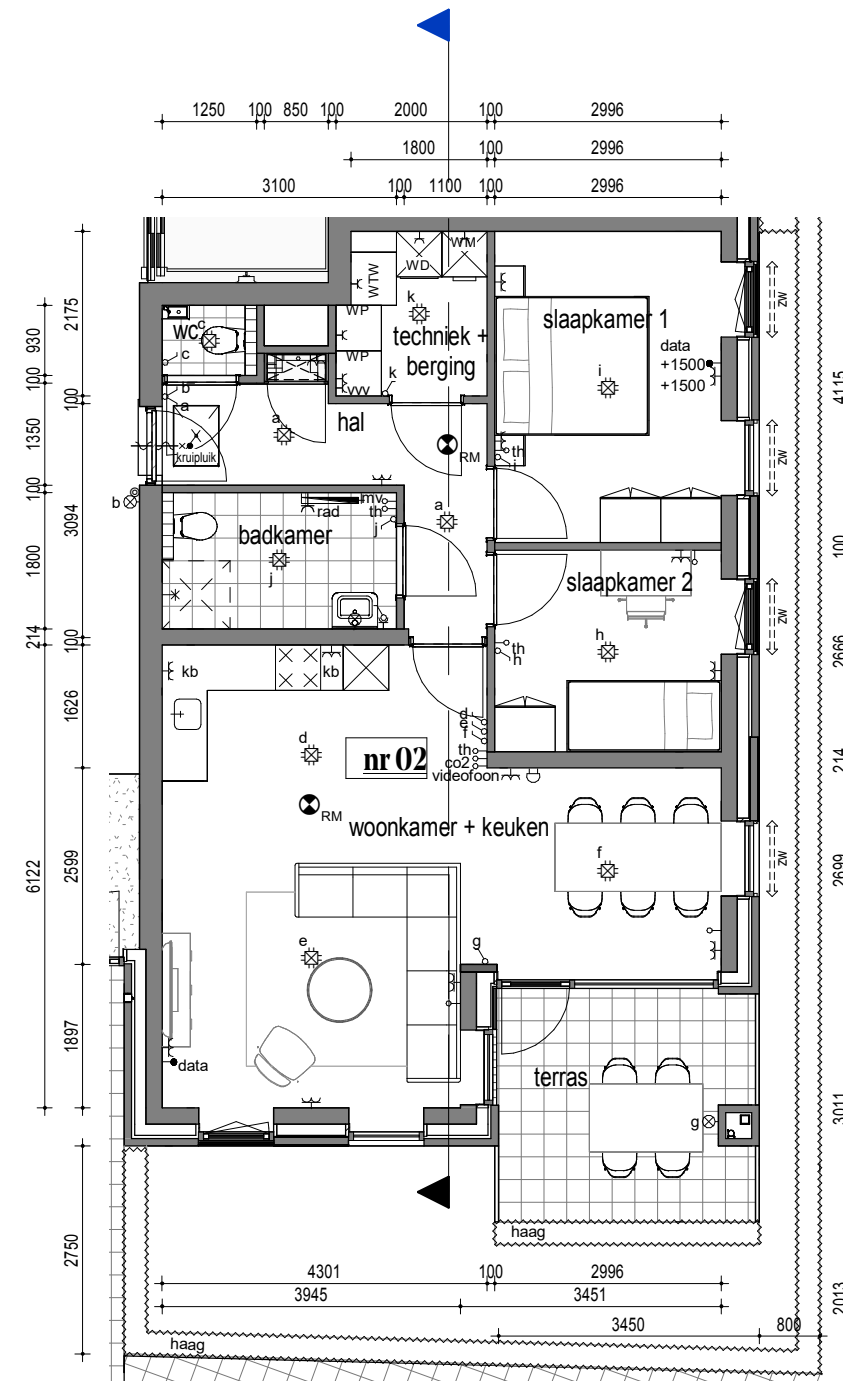
Plattegrond 1:100
