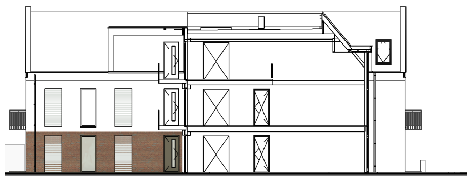
Linker zijgevel 1:250
